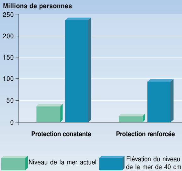
Figure 3-6 : Adaptation et nombre annuel moyen de personnes victimes d'inondations provoquées par des ondes de tempêtes côtières — projection pour les années 2080. Les deux barres de gauche représentent le nombre annuel moyen de personnes qui devraient être victimes d'inondations provoquées par des ondes de tempêtes côtières en 2080 pour le niveau de la mer actuel et pour une élévation du niveau de la mer de ~40 cm, en supposant une protection côtière inchangée par rapport à la situation actuelle, et une augmentation de population moyenne. Les deux barres de droite représentent la même chose, mais supposent une amélioration de la protection côtière proportionnelle à la hausse du PIB.
