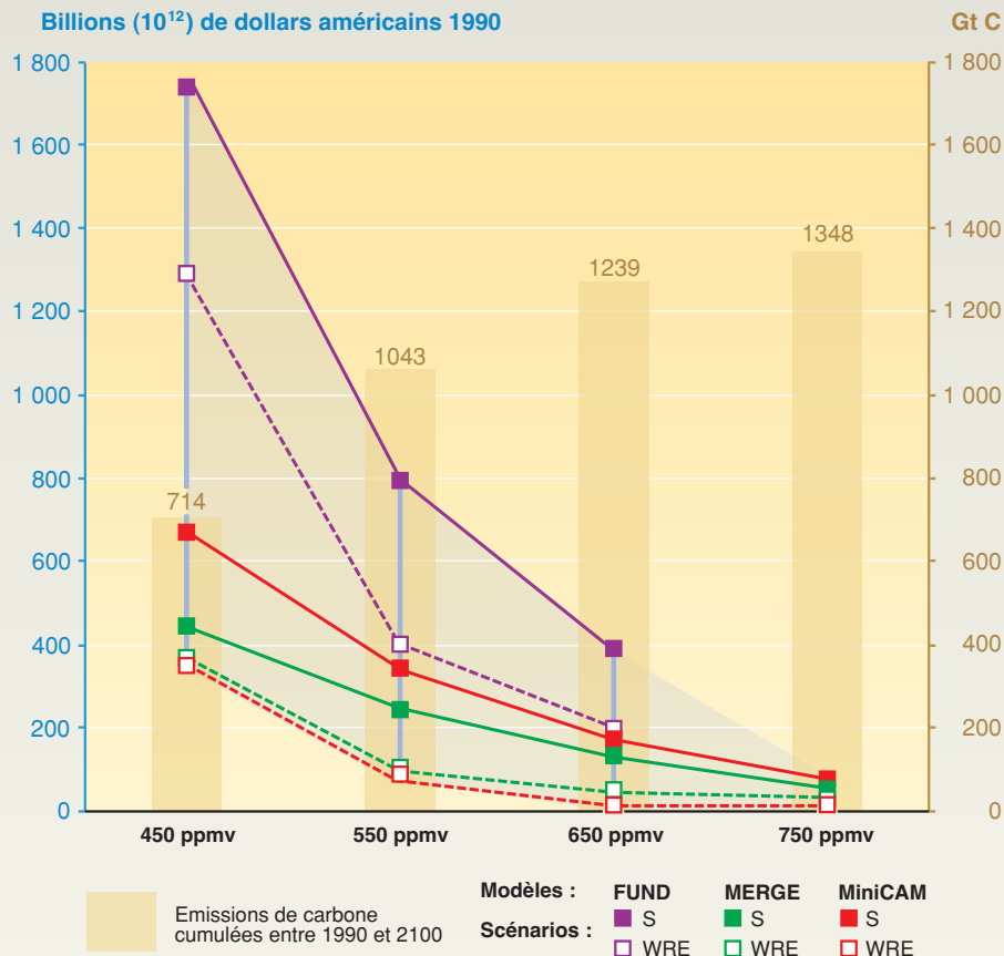
Figure 7-3 : Les coûts d'atténuation (dollars américains 1990, valeur actualisée à 5 % par an pour la période 1990–2100) de la stabilisation des concentrations de CO 2 entre 450 et 750 ppmv sont calculés à l'aide de trois modèles mondiaux, basés sur différents niveaux de références dépendant des modèles. Les incidences prévues des changements climatiques ne sont pas incluses. Dans chaque cas, les coûts ont été calculés à partir de deux chemins d'émissions pour atteindre l'objectif prescrit : S (intitulé chemins d'émissions GTI dans le TRE du GTIII) et WRE décrit dans la réponse à la Question 6. Les barres représentent les émissions de carbone cumulé entre 1990 et 2100. Les futures émissions cumulées jusqu'à ce que soit atteint un plafond budgétaire pour le carbone sont représentées au-dessus des barres en Gt C.
